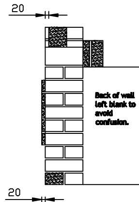
END ELEVATION
