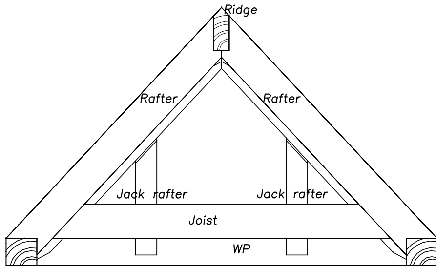
End Elevation
