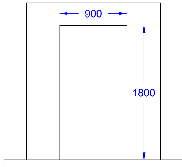
ELEVATION A
