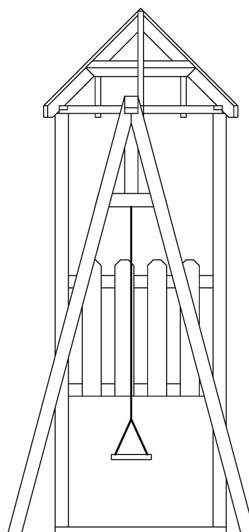
END ELEVATION
