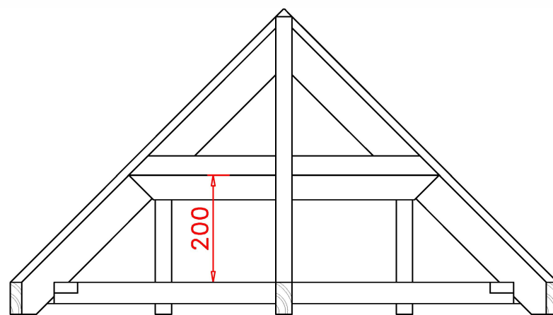
END ELEVATION
