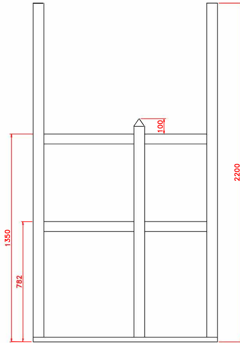
ELEVATION
