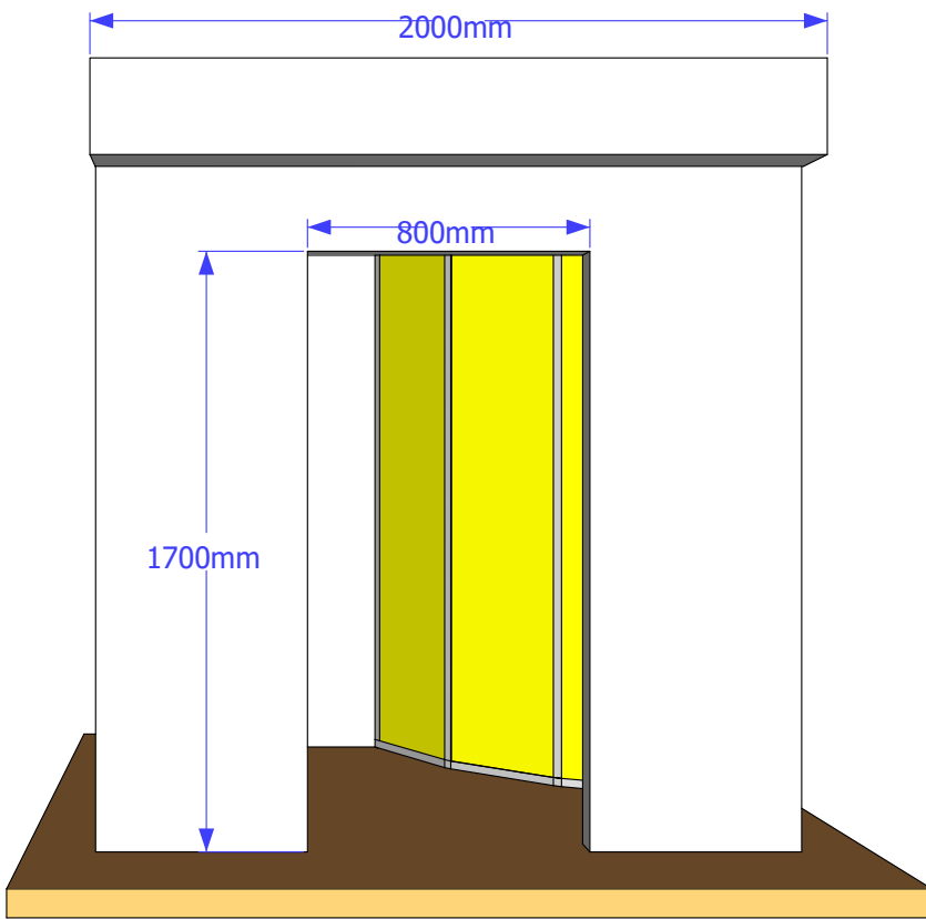
Elevation A
